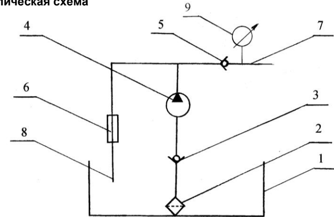
Гидравлическая схема
